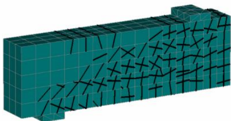
Gambar 11. Pola retak balok dengan sudut tulangan sengkang 50°
