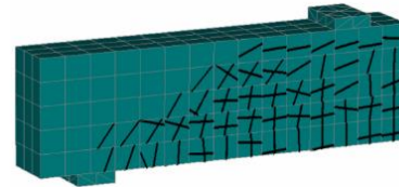
Gambar 13. Pola retak balok dengan sudut tulangan sengkang 70°
