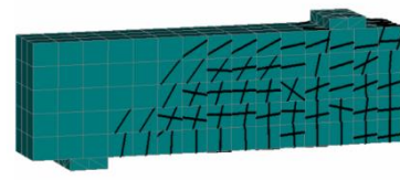
Gambar 12. Pola retak balok dengan sudut tulangan sengkang 60°
