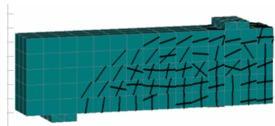
Gambar 14. Pola retak balok dengan sudut tulangan sengkang 90°
