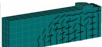
Gambar 16. Pola retak balok dengan sudut tulangan sengkang 120°
