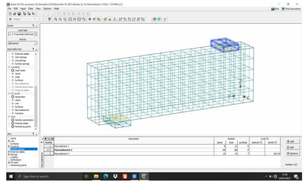
Gambar 6. Tampak balok setelah di FE Mesh
