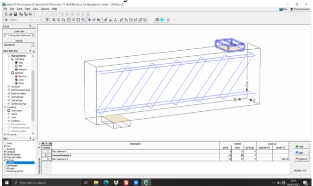
Gambar 5. Penulangan balok beton
