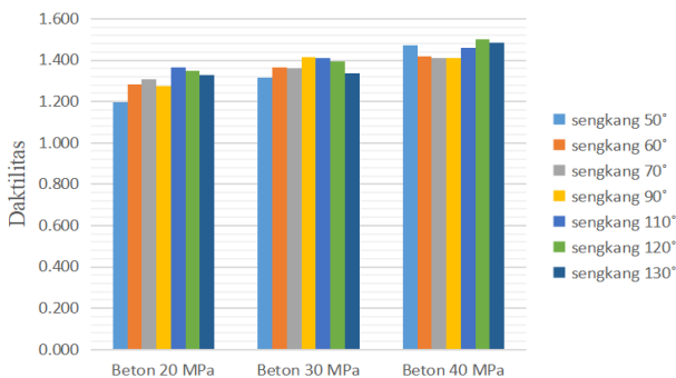
Gambar 10. Hasil nilai daktilitas balok beton bertulang
